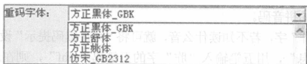
图 3-11 重码字体
